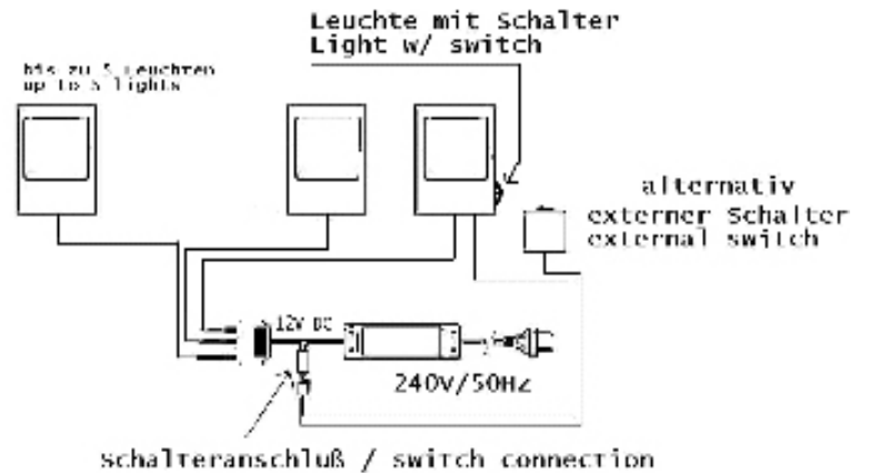
Anschlussschema SET mit Hauptschalter wiring diagram SET w/ main switch
